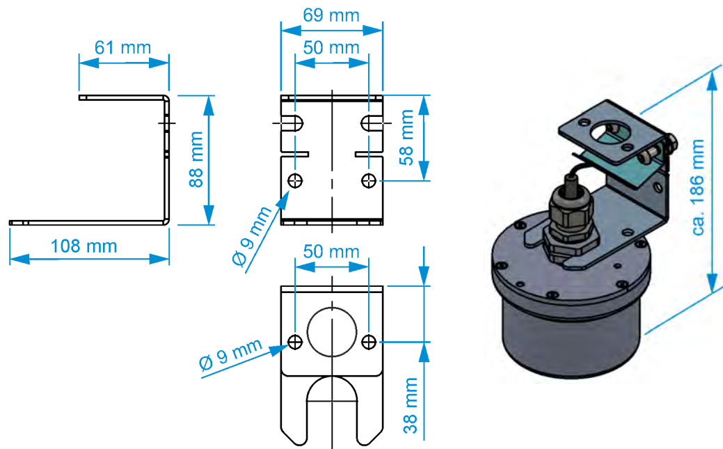
Abb. 24-3 Variante 2: An senkrechter Wand / an Decke mit Befestigungswinkel
