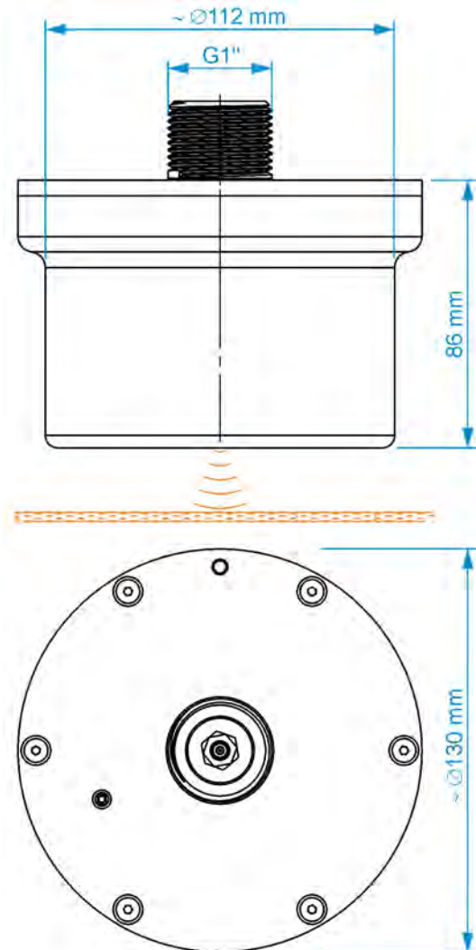
Abb. 15-2 Gehäuse
