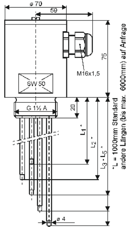
Hängeelektrode Xfach hier 3fach (IP54)
