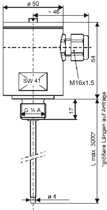
Stabelektrode 1fach (IP54)
