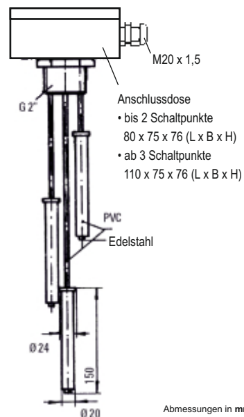
Hängeelektrode Xfach hier 3fach (IP54)
