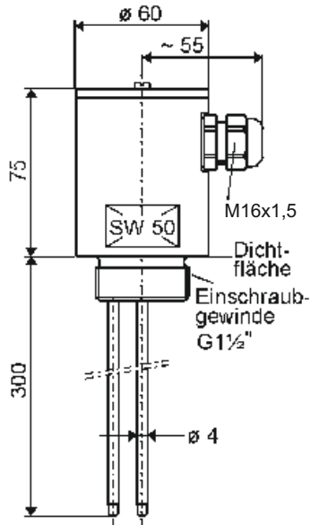
Stabelektrode 2fach § 19 WHG (IP65)
