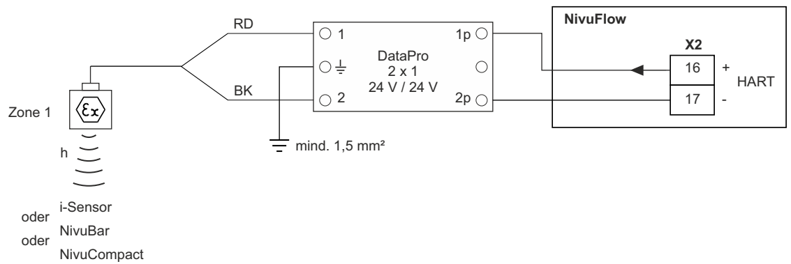
Abb. 17-10 Überspannungsschutz externe Füllstandsmessung
