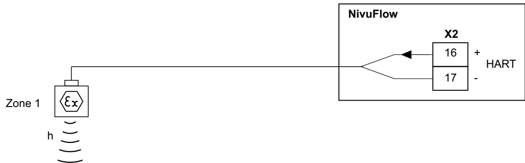
Abb. 17-5 Anschluss 2-Leiter-Sensor Ex zur Füllstandmessung
