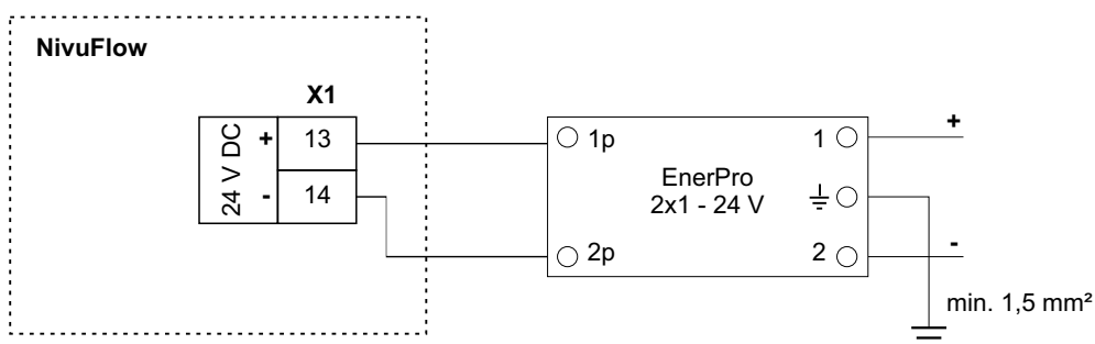
Abb. 17-8 Überspannungsschutz für Spannungsversorgung DC allgemein
