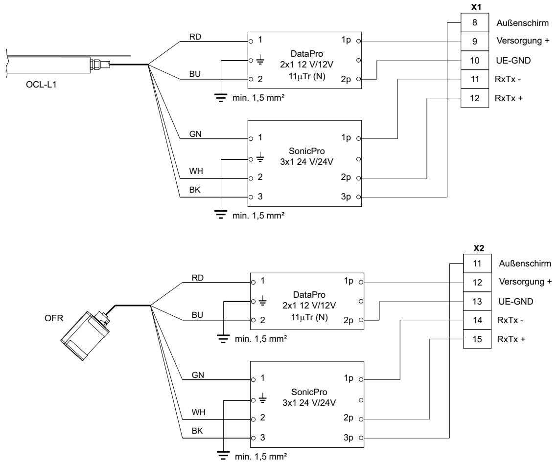
Abb. 17-9 Überspannungsschutz der Sensoren für R1
