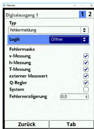
Abb. 23-32 Fehlermaske
