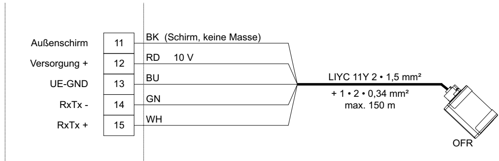
Abb. 17-4 Anschluss Radarsensor, Typ OFR
