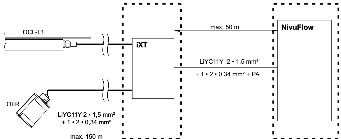
Abb. 17-1 Anschluss Ex-Trennmodul iXT an NivuFlow über Standardkabel
