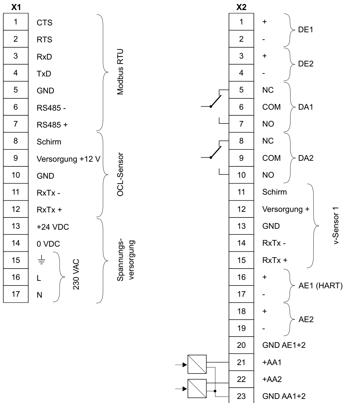
Abb. 18-1 Allgemeiner Anschlussplan, NivuFlow 550, Typ R1
