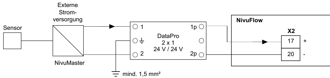
Abb. 17-11 Überspannungsschutz Analogeingang von ext. Messumformer
