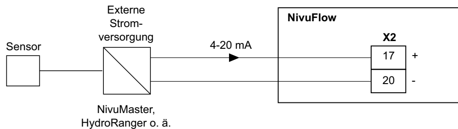
Abb. 17-6 Anschluss externe Füllstandsmessung
