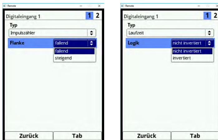
Abb. 23-28 Umstellmöglichkeiten Logik
