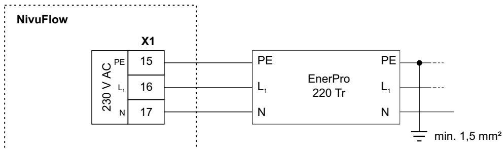
Abb. 17-7 Überspannungsschutz für Spannungsversorgung AC allgemein
