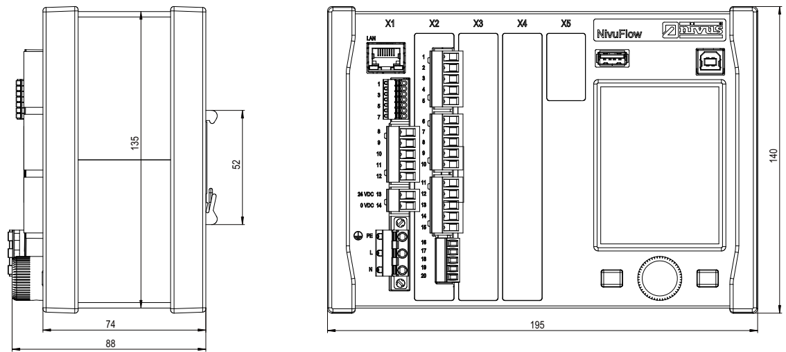
Abb. 9-2 Maße Messumformer NivuFlow 550
