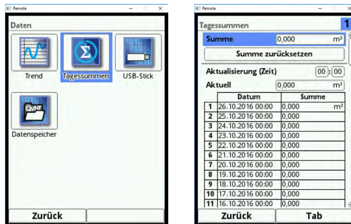
Abb. 24-3 Auswahl Tagessummen
