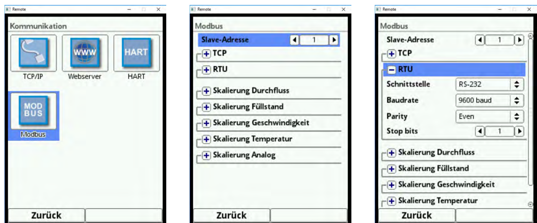
Abb. 26-2 Modbus
