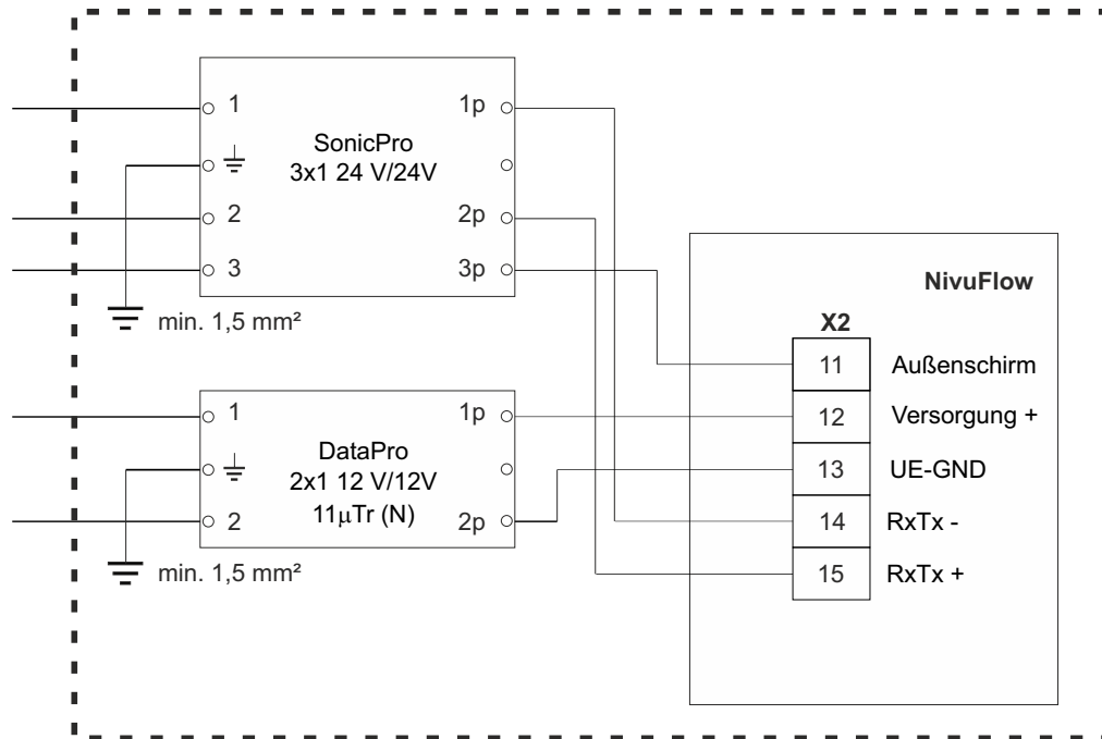
Abb. 17-12 Überspannungsschutz iXT an NivuFlow 550
